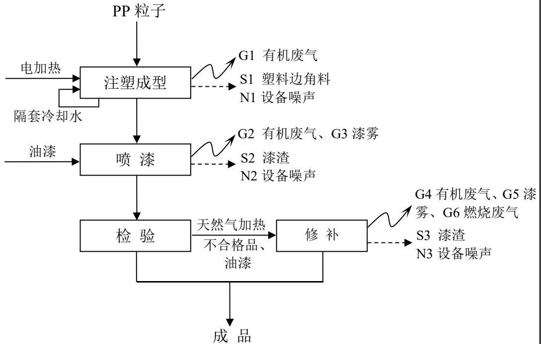
图 2-9 汽车饰件生产工艺及产污环节流程图
